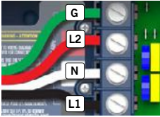
240 V (4 wires)
