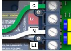
120 V (*3 wires)
